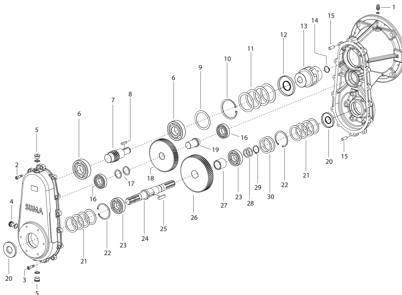
Abb. 4: Stirnradgetriebe Rührgigant FT - i=3,69 Spur gearing Giantmix FT - i=3.69
