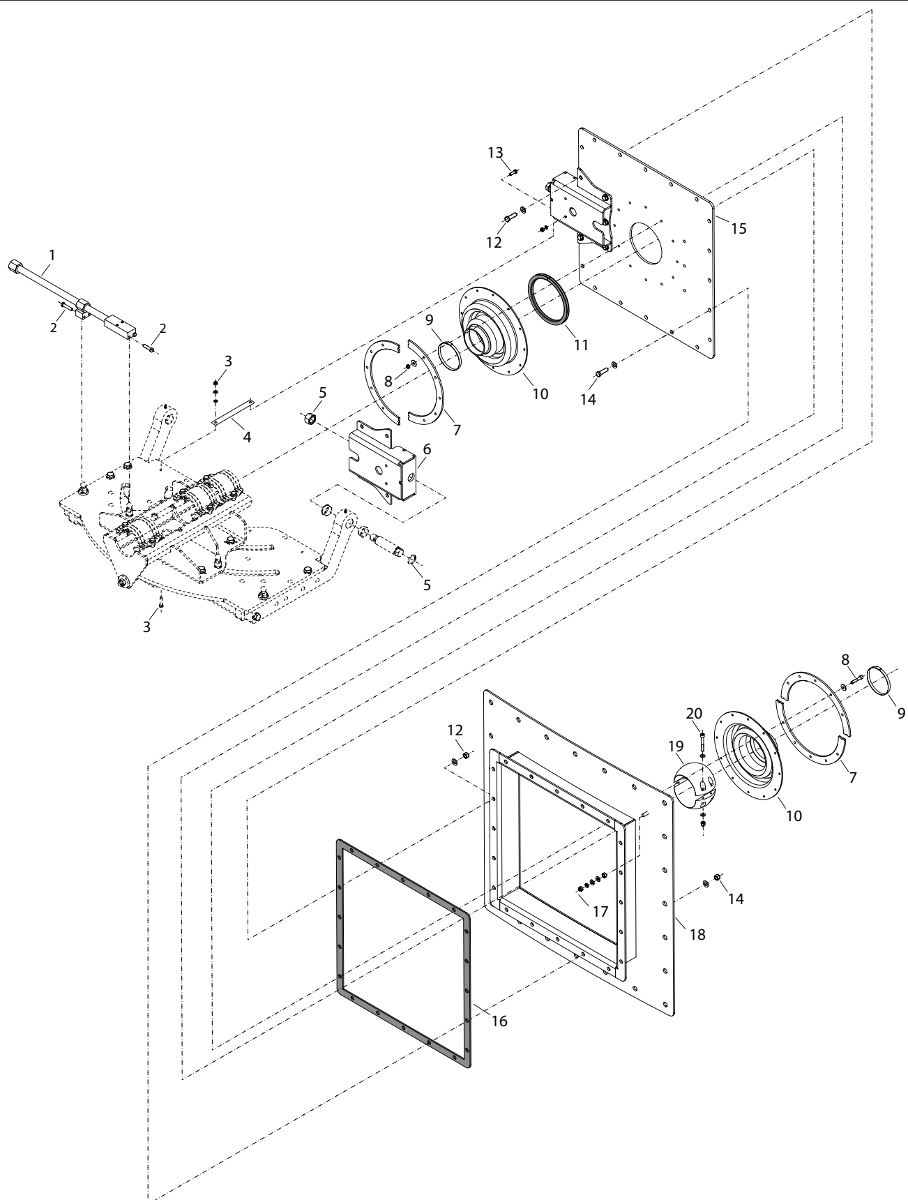
Abb. 6: Dichtplatte mit Schwenkeinrichtung Sealing plate with articulated frame
