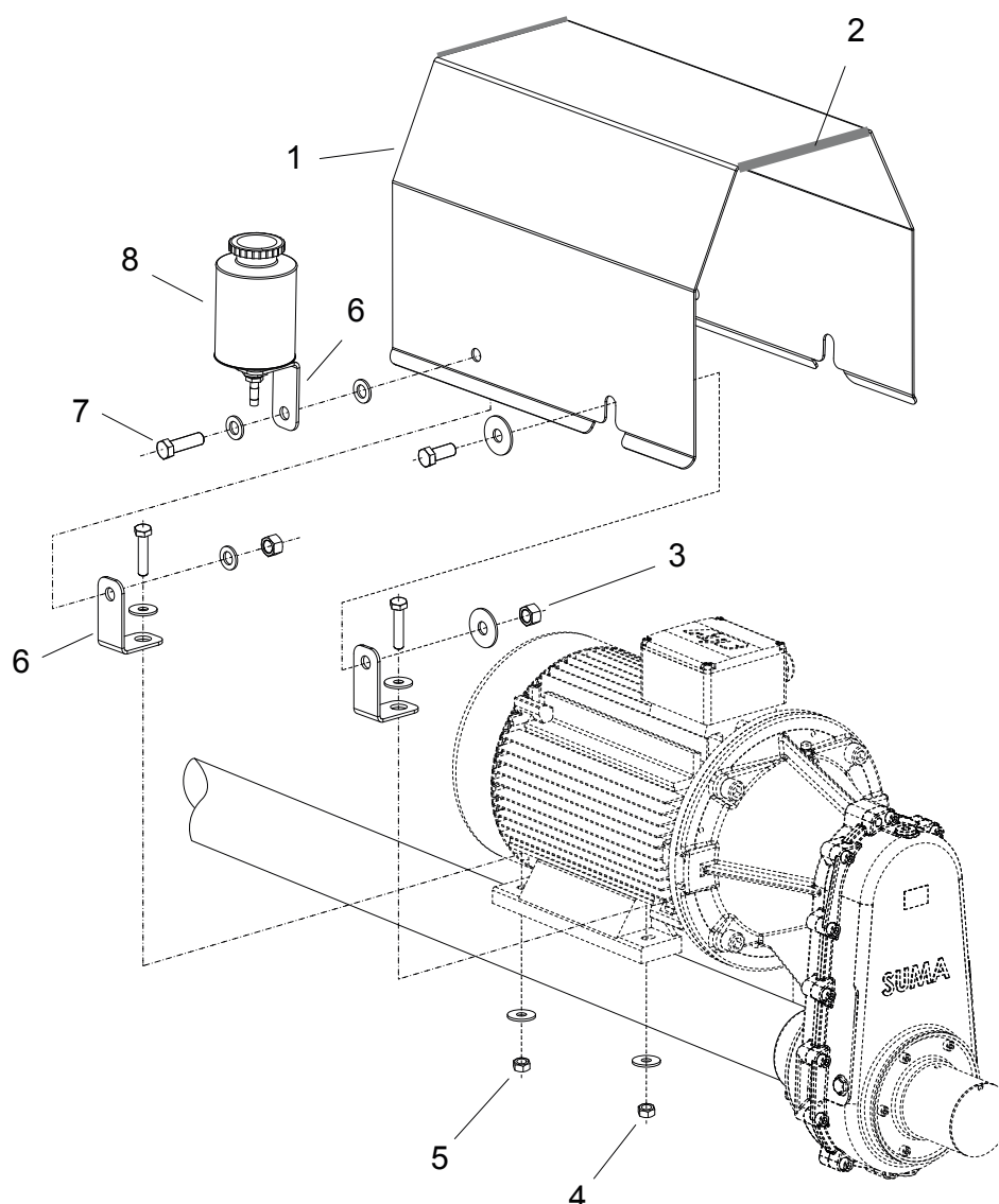
Abb. 14: Schutzhaube für Elektromotor (Option) Protective hood for electric motor (option)
