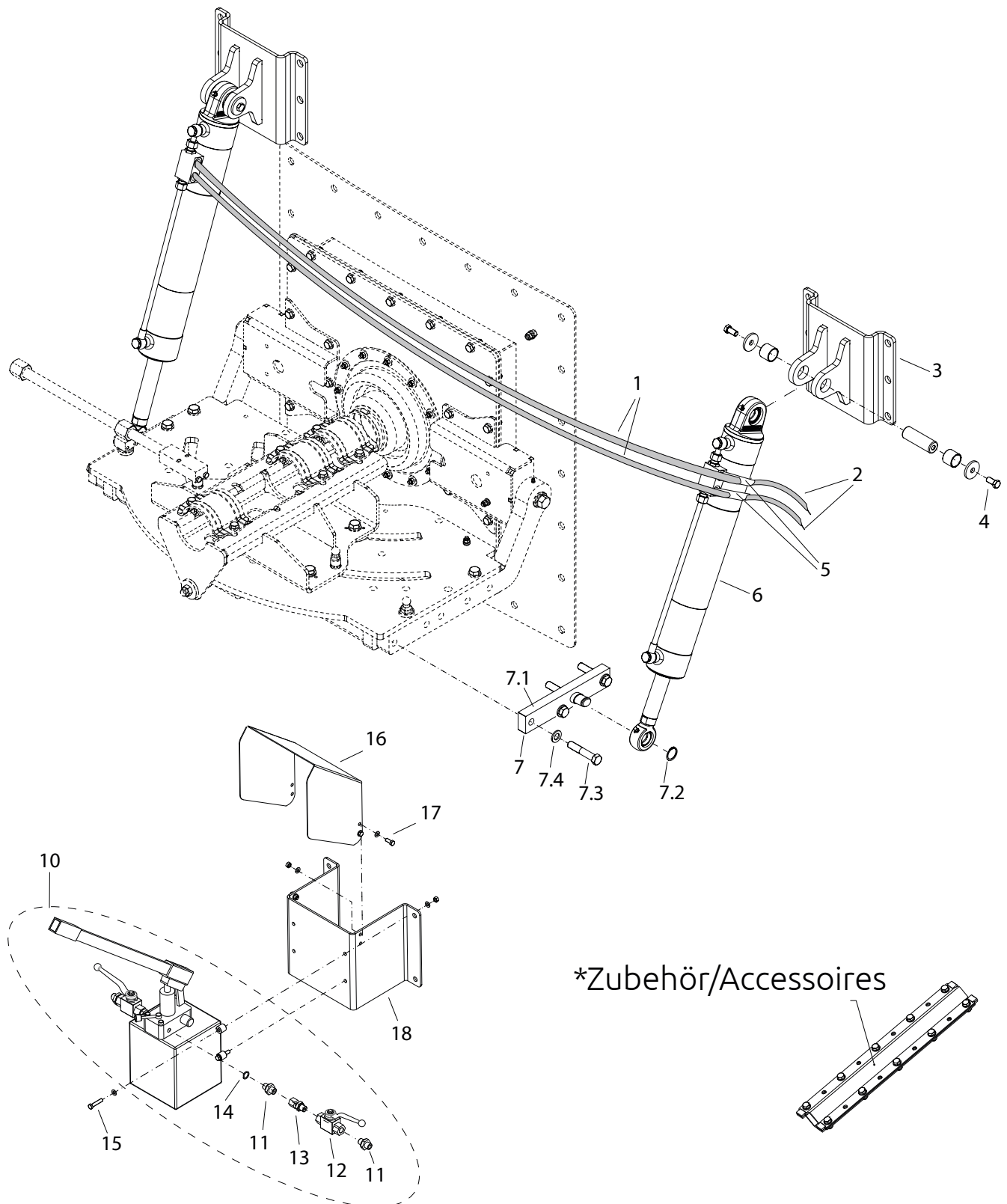
Abb. 13: Rührgigant FR SP mit Hydraulikzylinder oben Giantmix FR SP with hydraulic cylinder above
