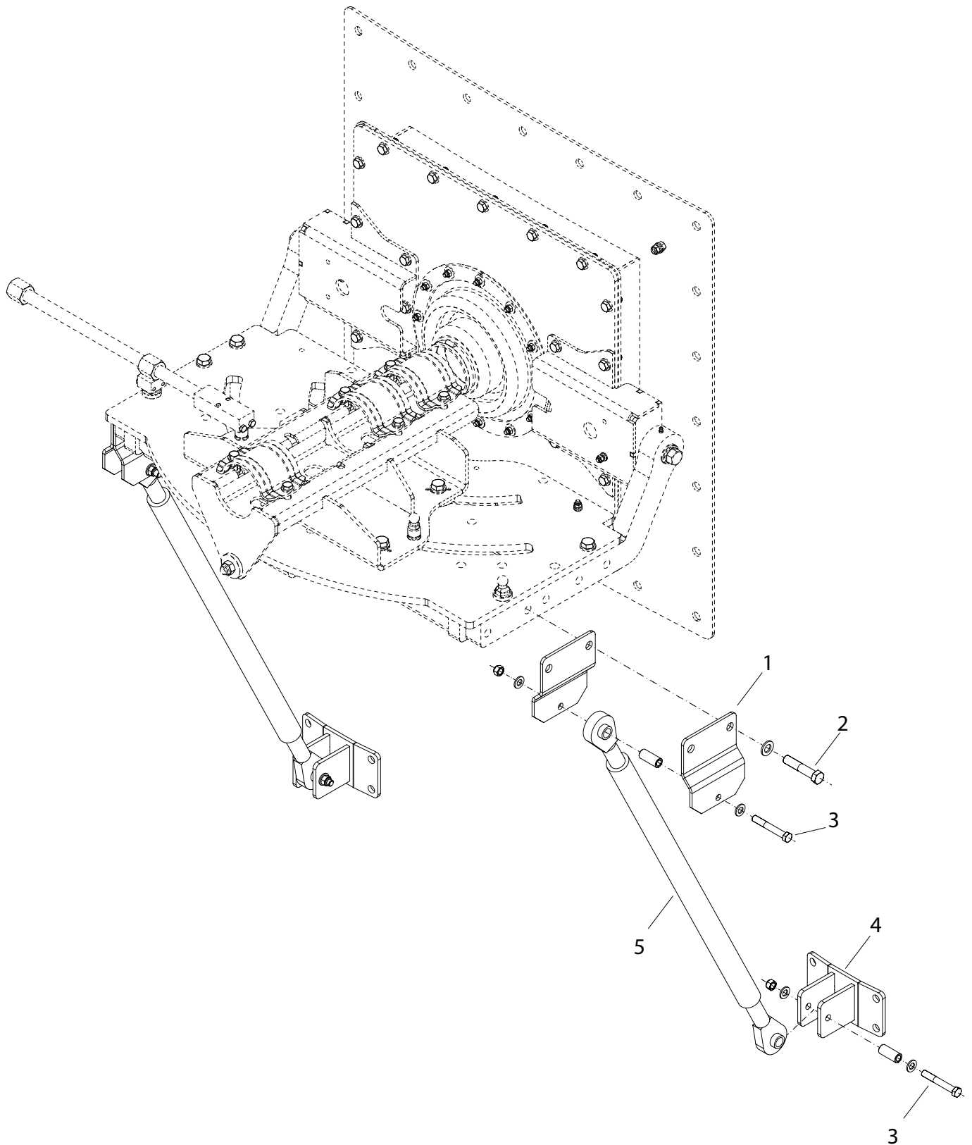
Abb. 8: Rührgigant FR SP mit Oberlenker unten Giantmix FR SP with upper link below
