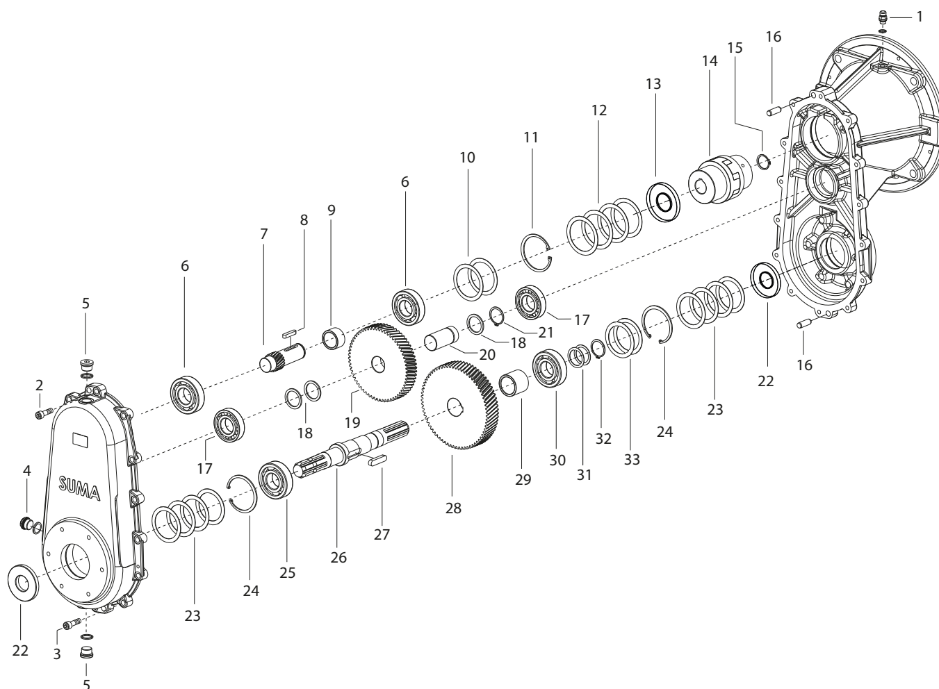
Abb. 5: Stirnradgetriebe Rührgigant FT - i=5,31 (LL) Spur gearing Giantmix FT - i=5,31 (LL)
