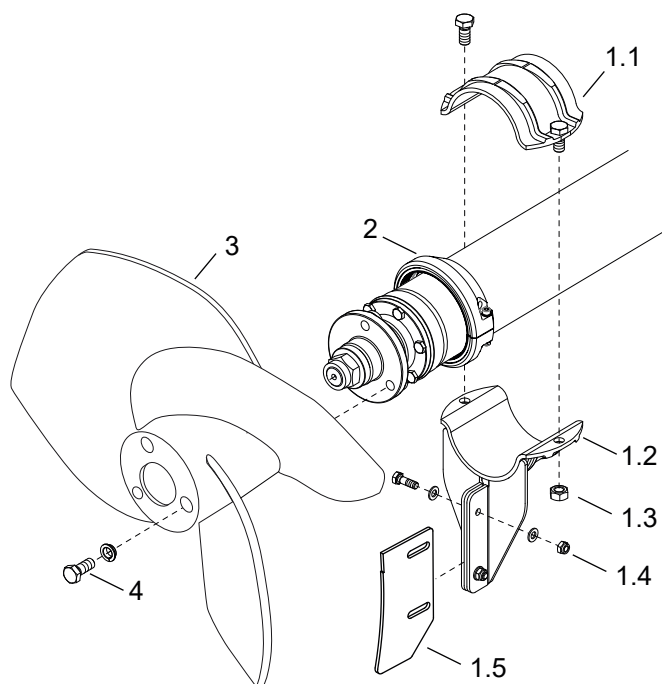
Abb. 1: Rohrende mit Rührflügel und Abstreifer Tube end with propeller and scraper
