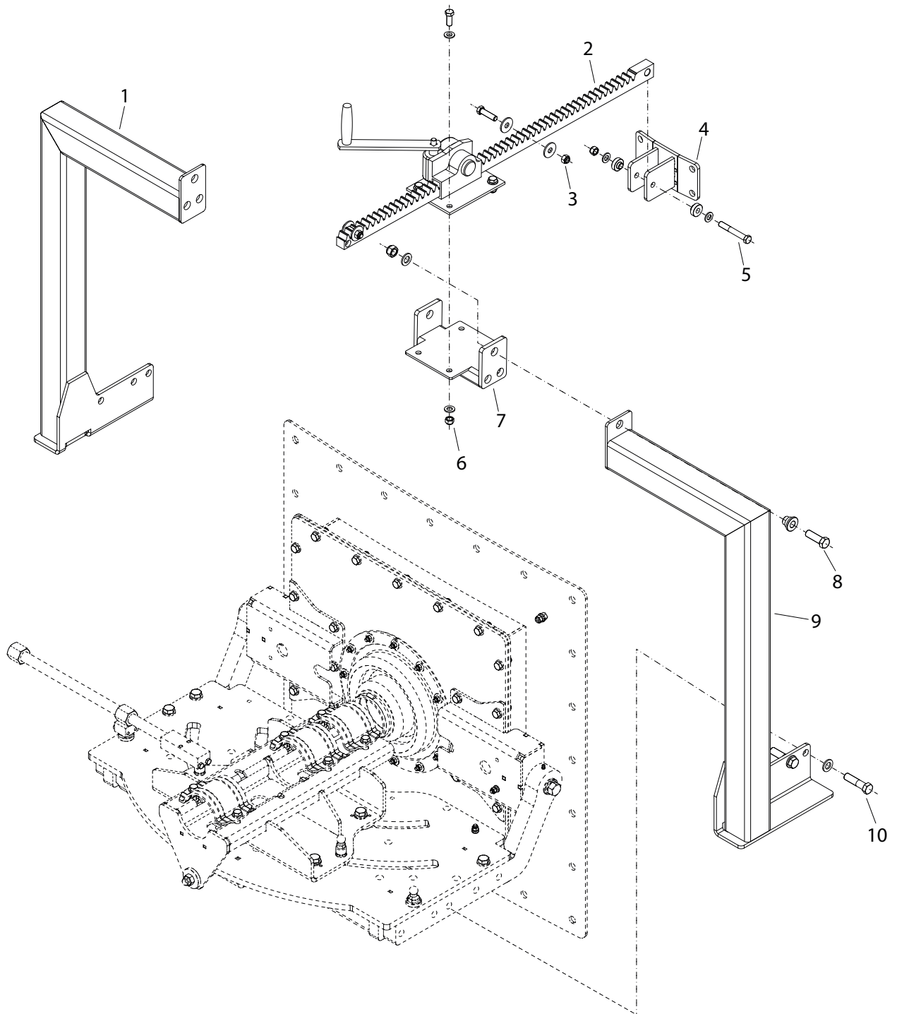
Abb. 11: Rührgigant FR SP mit Zahnstange oben Giantmix FR SP with pinion rack above
