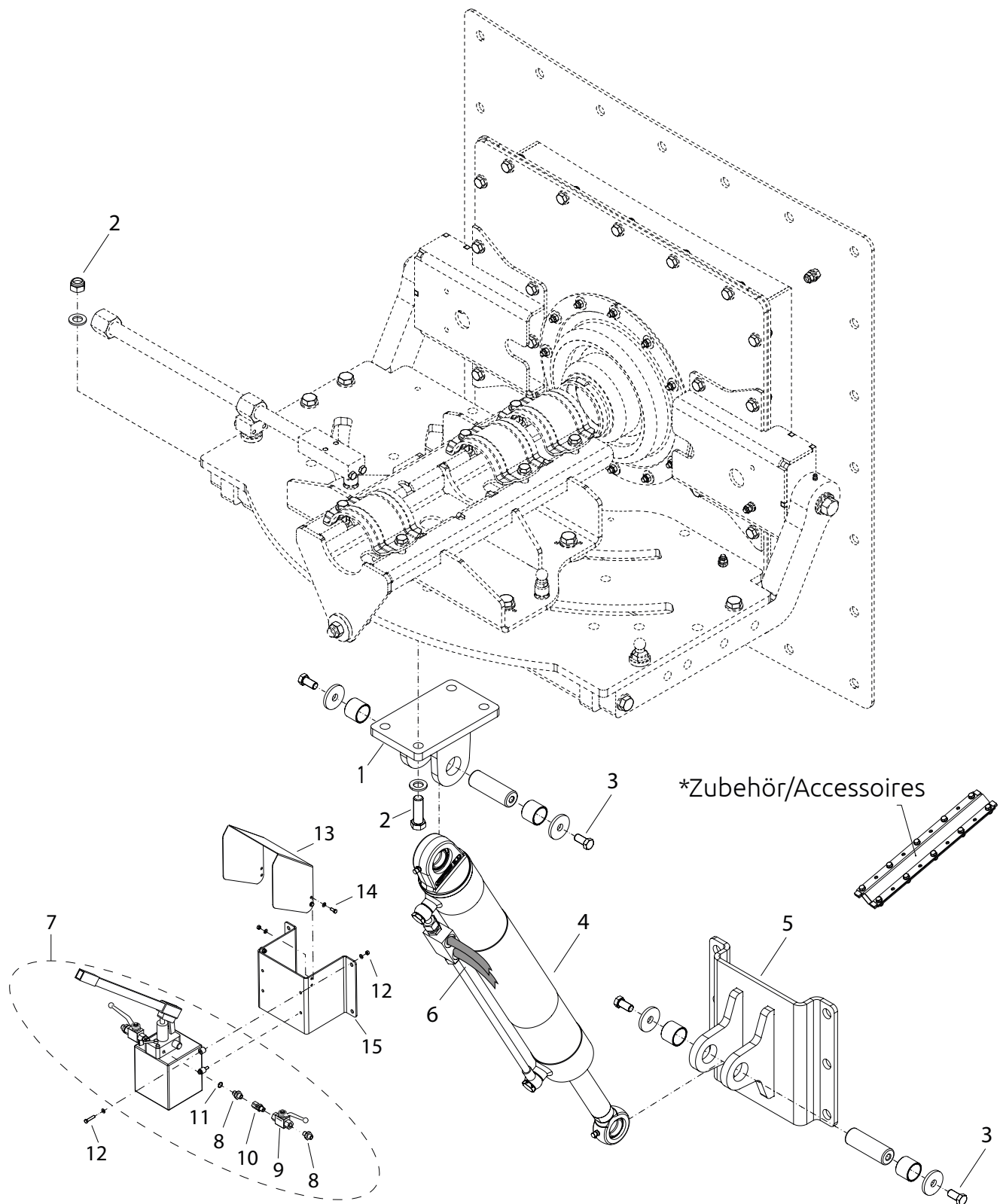
Abb. 12: Rührigigant FR SP mit Hydraulikzylinder unten Giantmix FR SP with hydraulic cylinder below
