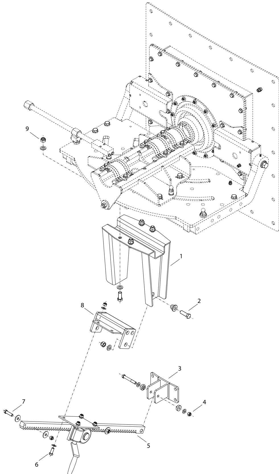
Abb. 10: Rührgigant FR SP mit Zahnstange unten Giantmix FR SP with pinion rack below
