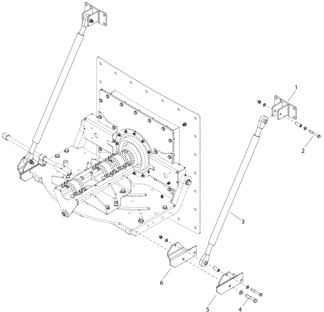
Abb. 9: Rührgigant FR SP mit Oberlenker oben Giantmix FR SP with upper link above
